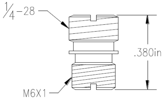
M6x1 Stud
